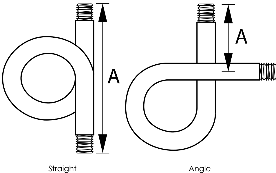
1/4" I.P.S Syphons
